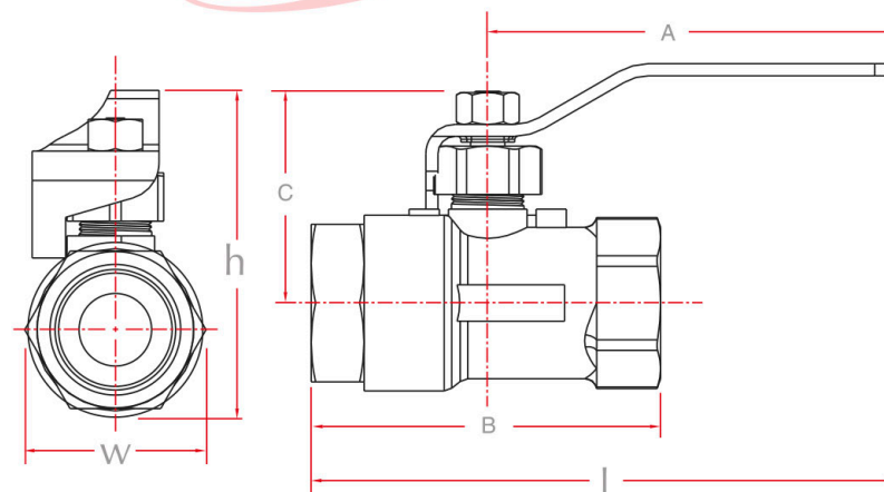
Dimensiones • Dimensions
